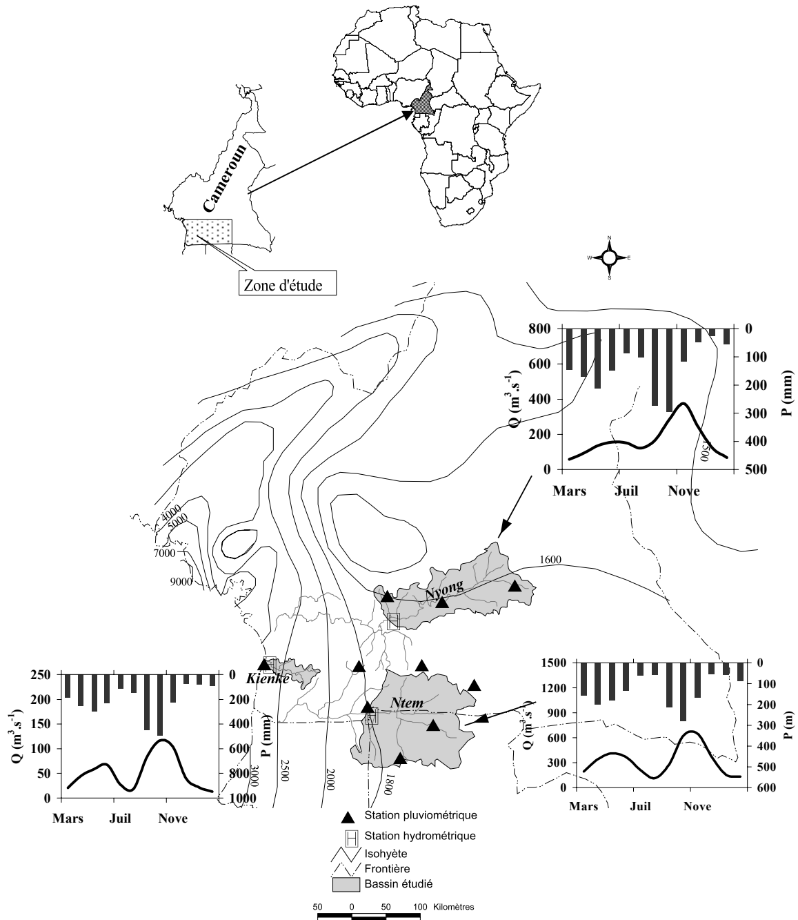
Fig. 1 Profils saisonniers des pluies et des écoulements sur trois bassins du sud-Cameroun.
