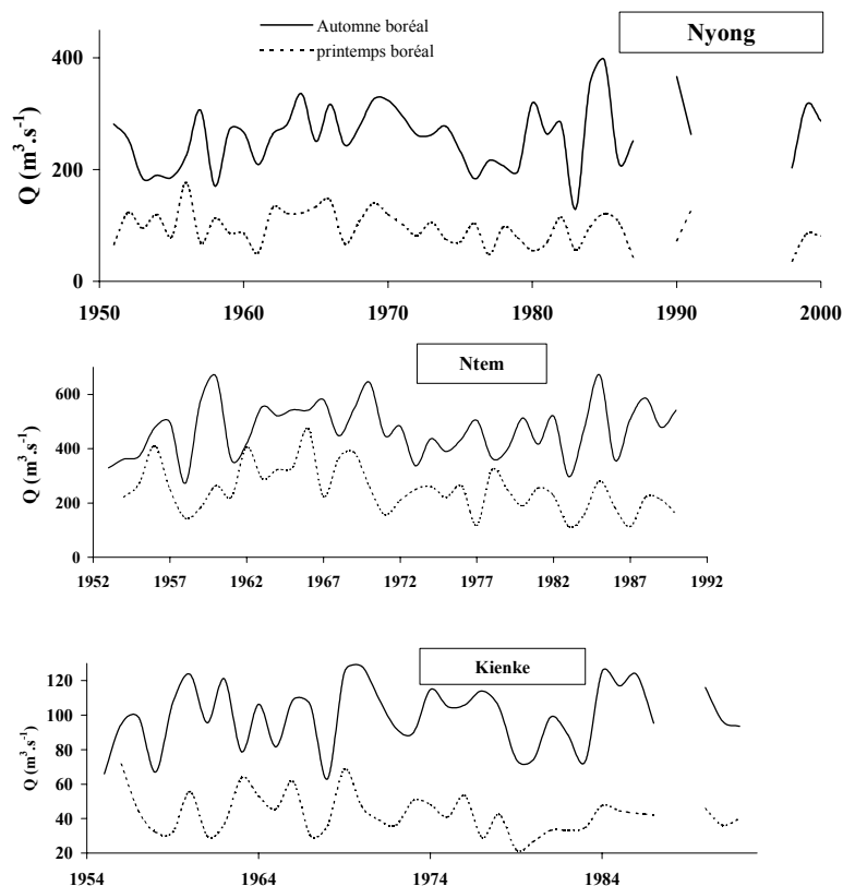
Fig. 3 Evolution des modules saisonniers des crues de printemps et d'automne sur la période 1951-1987.
