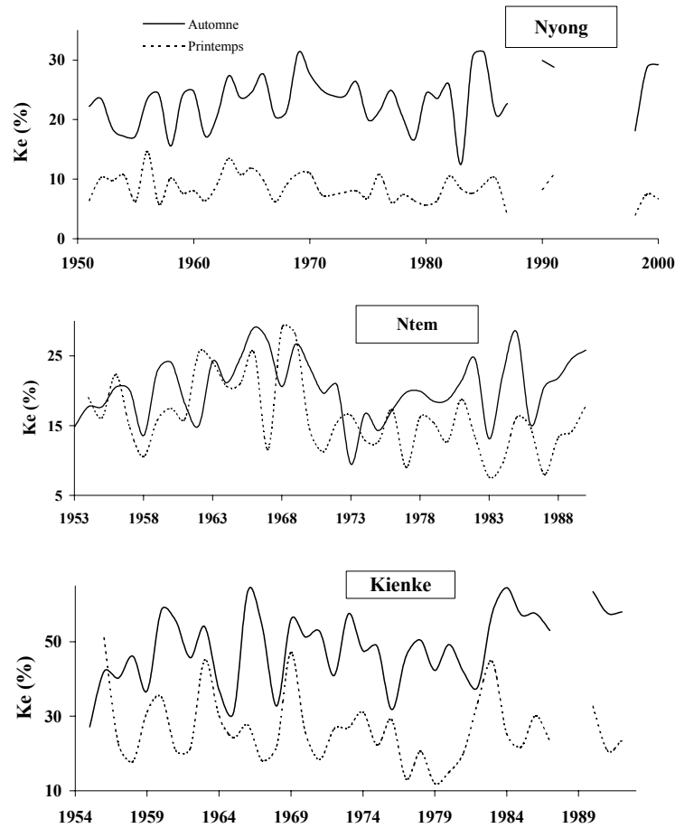
Fig. 4 Evolution des coefficients d'écoulements des crues de printemps et d'automne.
