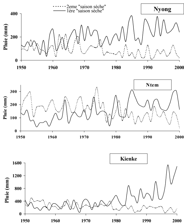
Fig. 2 Evolution de la pluviométrie des “saisons sèches” en zone équatoriale camerounaise sur la période 1950–2000.
